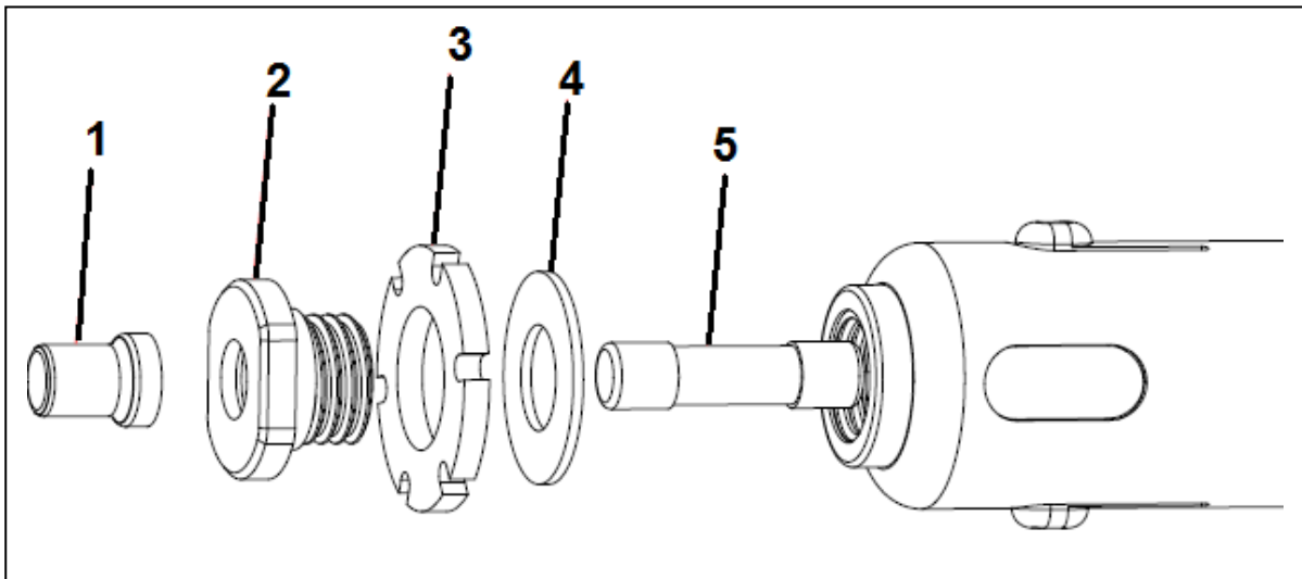
1. Spitze, 2. Schraubverschluss, 3. Silikonring, 4. Dichtung, 5. Sicherung
